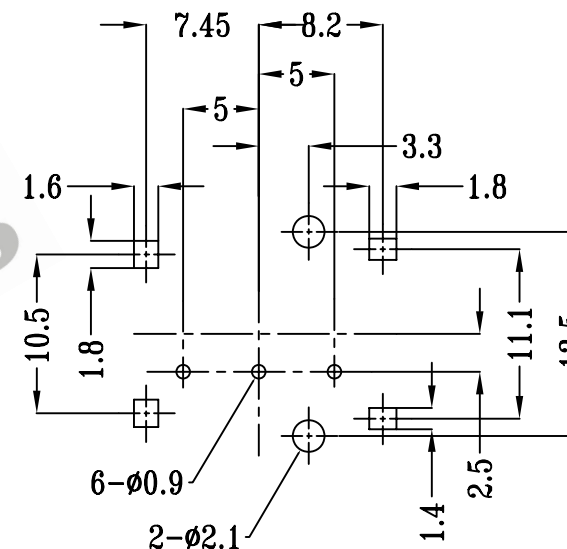
P.C.B LAYOUT
